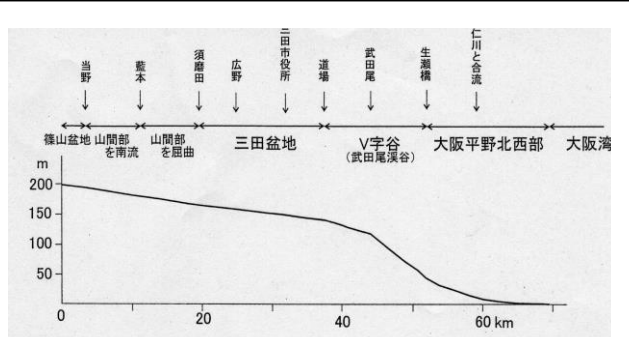
図6 武庫川の河川縦断面図。
