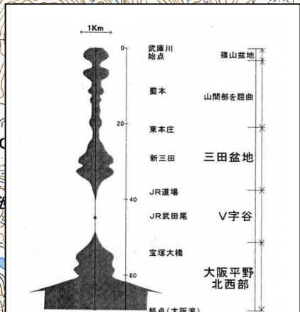
図3 武庫川の沖積低地の分布幅。武庫川源流部に幅広い沖積低地が分布していること、三田盆地と大阪平野の間はV字谷が発達し、沖積低地が見られないことに注意。図2の河川縦断面図を参照。
