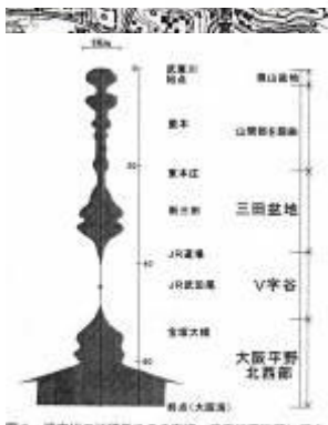
図3 武庫川の沖積盆地の分布概観。武庫川流域部に幅広い沖積盆地が分布していること、三田盆地と大阪平野の間はV字谷が発達し、沖積盆地が変られないことに注意。図2の河川断面図を参照。
